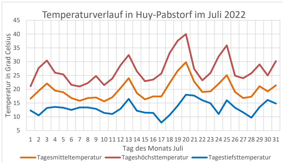
Abbildung 1: Verlauf der Tagesmittel-, Tageshöchst- und Tagestiefsttemperatur an der Wetterstation Huy-Pabstorf im Juli 2022
