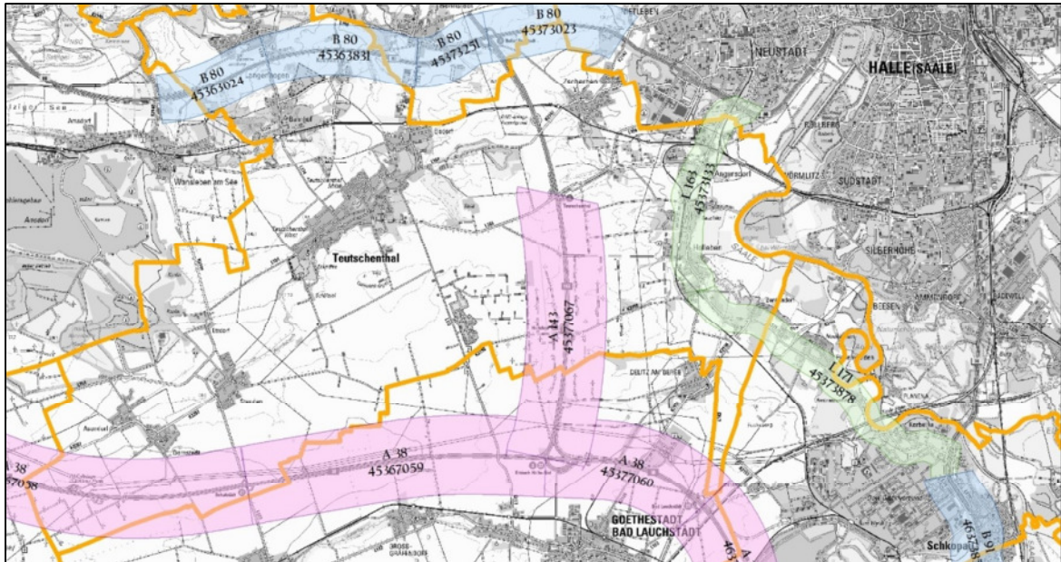
Abb. 4: Übersichtskarte mit dem Kartierungsumfang für TEUSCHENTHAL
