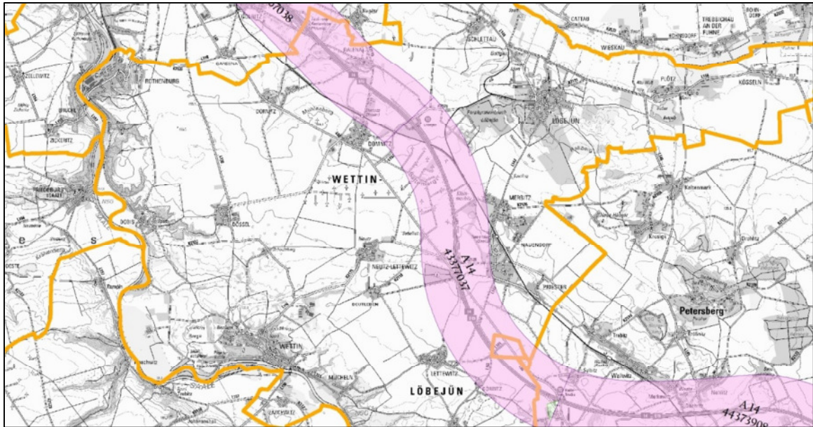
Abb. 4: Übersichtskarte mit dem Kartierungsumfang für WETTIN-LÖBEJÜN
